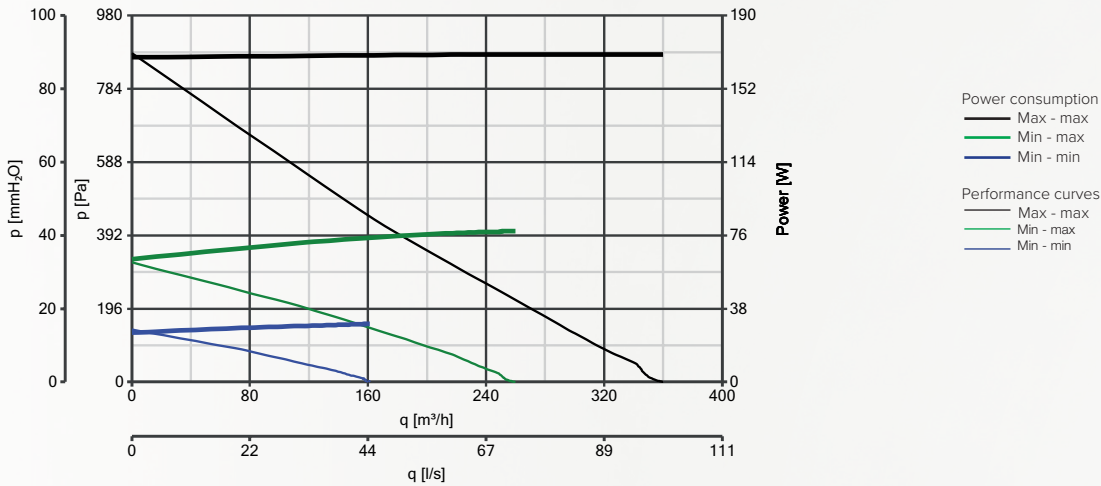
VORT HR 350 AVEL
